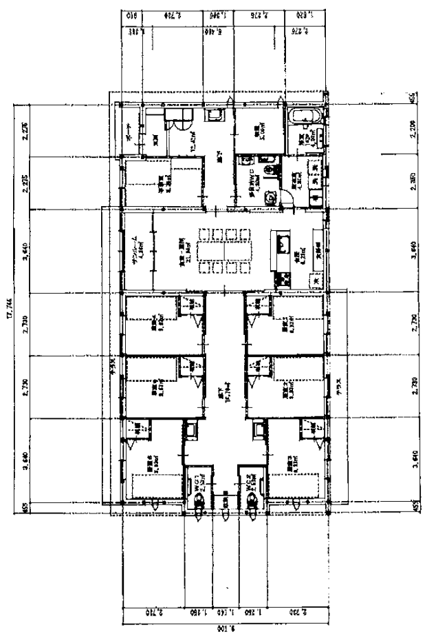
平面図 (北を上に示す)
